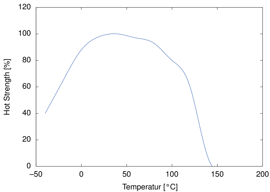
Abbildung 2: Hot Strength (%RT Festigkeit, getestet bei Temperatur)
