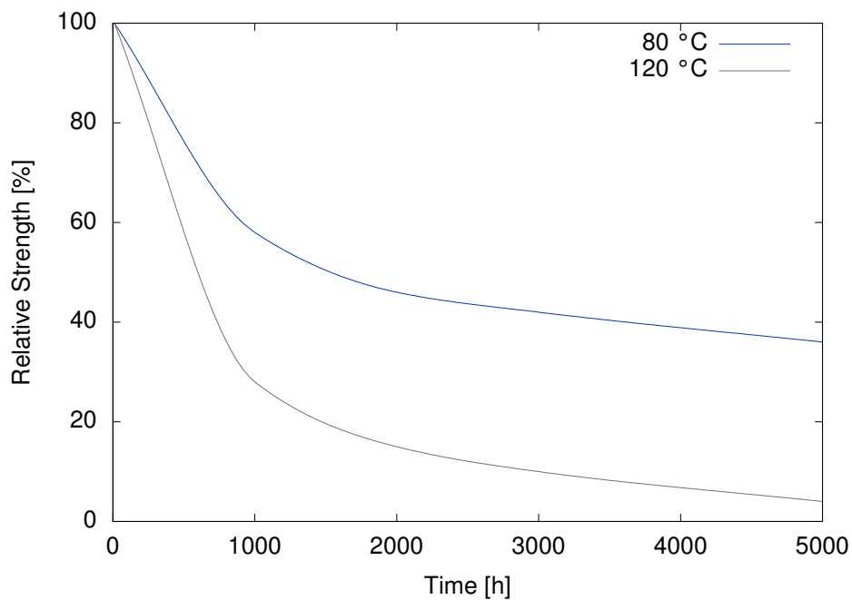
Abbildung 4: Alterung an Stahl (getestet bei 20 °C)
