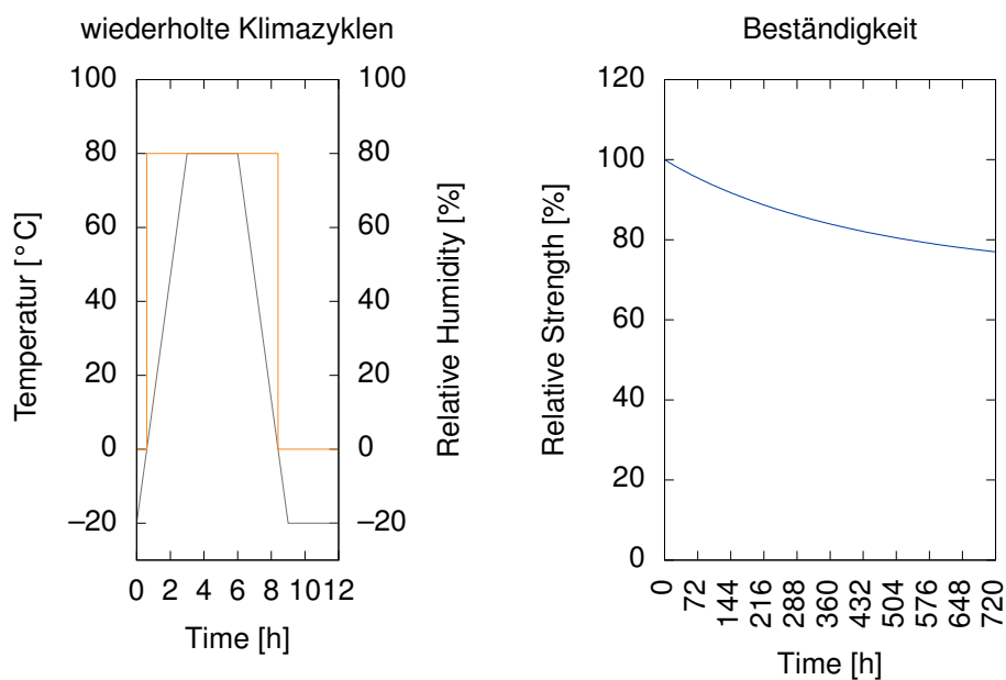
Abbildung 5: Beständigkeiten nach Wechselklimalagerung
