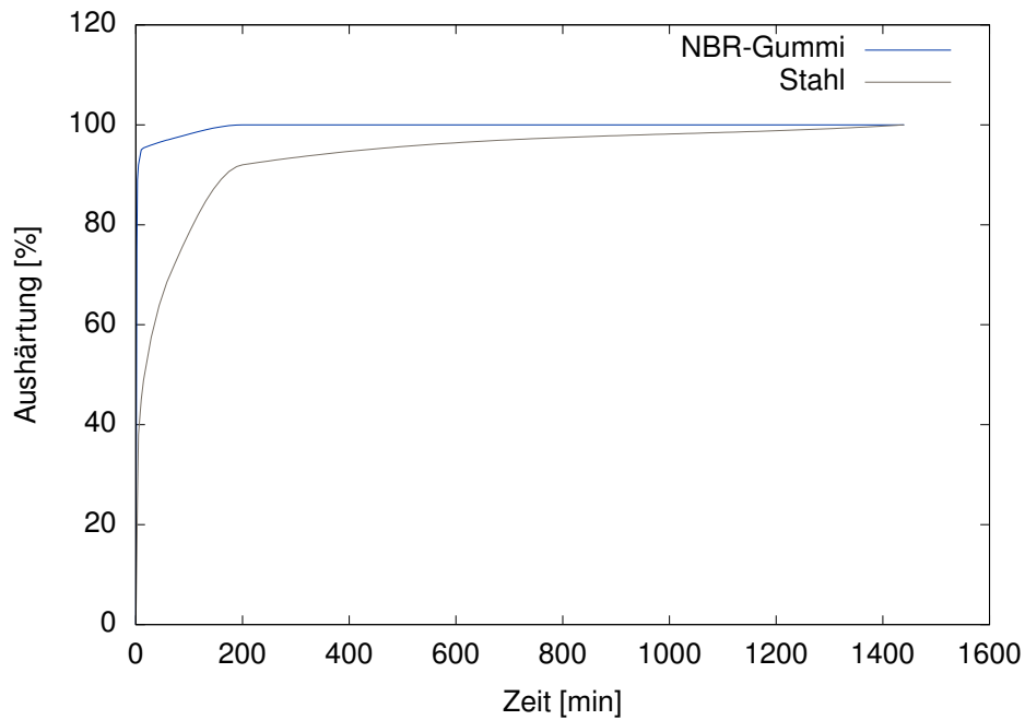
Abbildung 3: Zeit bis zur vollständigen Aushärtung
