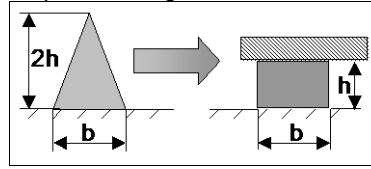
Abb. 1: Empfohlene Raupengeometrie
